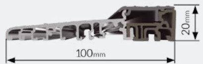
Drzwi Energooszczędne (pasywne) – grubość 100 mm – zawias widoczny
