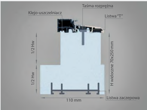
Drzwi standardowe – grubość 82 mm – zawias widoczny
