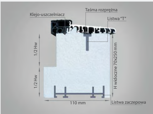
Drzwi Energooszczędne (pasywne) – grubość 100 mm – zawias widoczny
