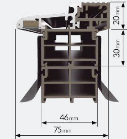
Drzwi standardowe – grubość 82 mm – zawias widoczny
